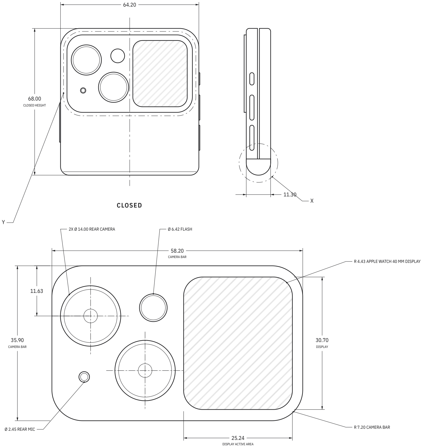
DETAIL Y · CAMERA BAR · SCALE 2:1
