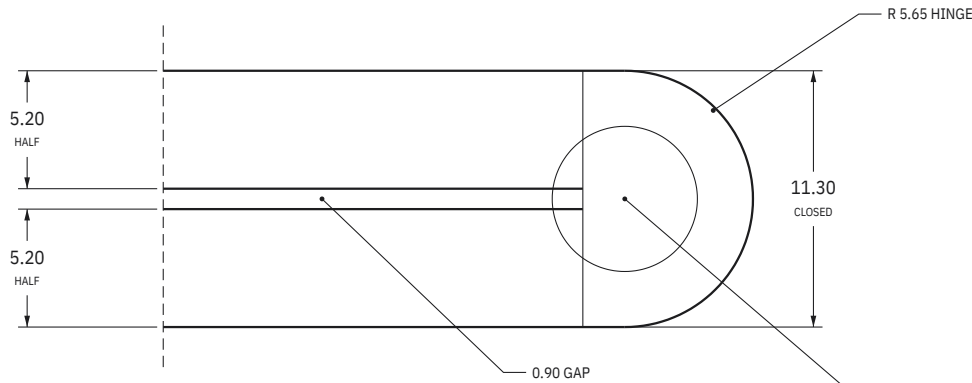
DETAIL X · HINGE · SCALE 3:1
